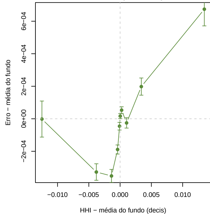
C) Dentro do fundo corr=0.06 (N=35.008)
