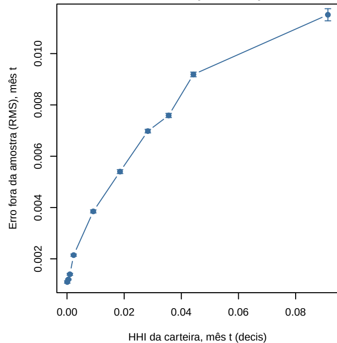
A) Contemporânea corr=0.48 (N=36.887)
